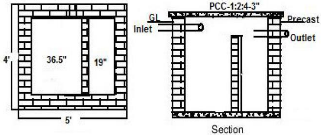
Septic Tank-Plan
